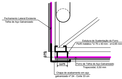
DETALHE A - Forro esc. 1:5
