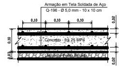
DETALHE B - Piso de Concreto esc. 1:5
